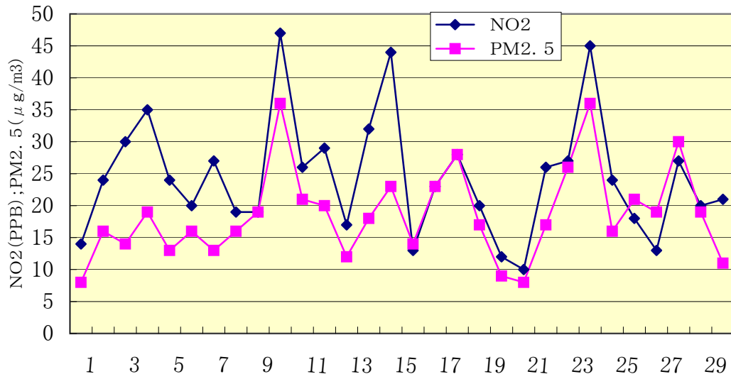
綾瀬測定局における日平均NO2とPM2.5の月間変動図 (2004年6月)
