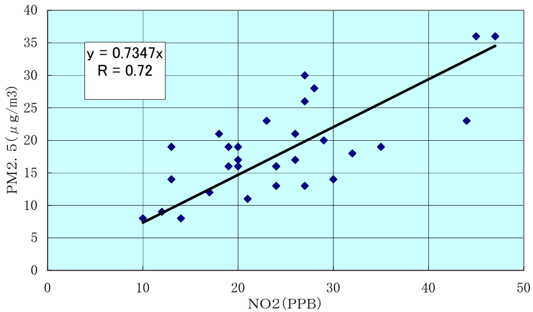
綾瀬一般測定局における日平均NO2とPM2.5の相関図 (2004年6月)
