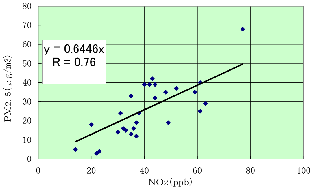
梅島自排局におけるNO2とPM2.5の相関図 (2006年10月)
