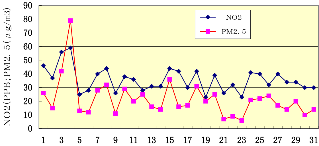
綾瀬一般測定局における日平均NO 2 とPM 2.5 の月間変動図 (2004年12月)
