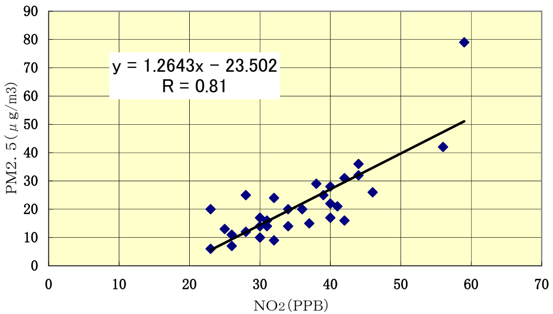
綾瀬一般測定局における日平均NO 2 とPM 2.5 の相関図 (2004年12月)
