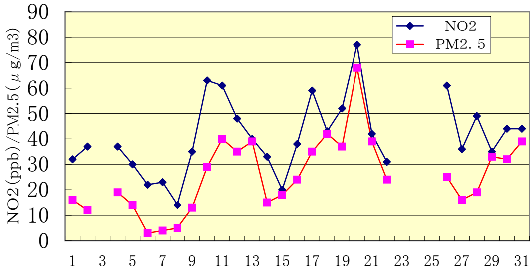
梅島自排局におけるNO2とPM2.5の月間変動図 (2006年10月)
