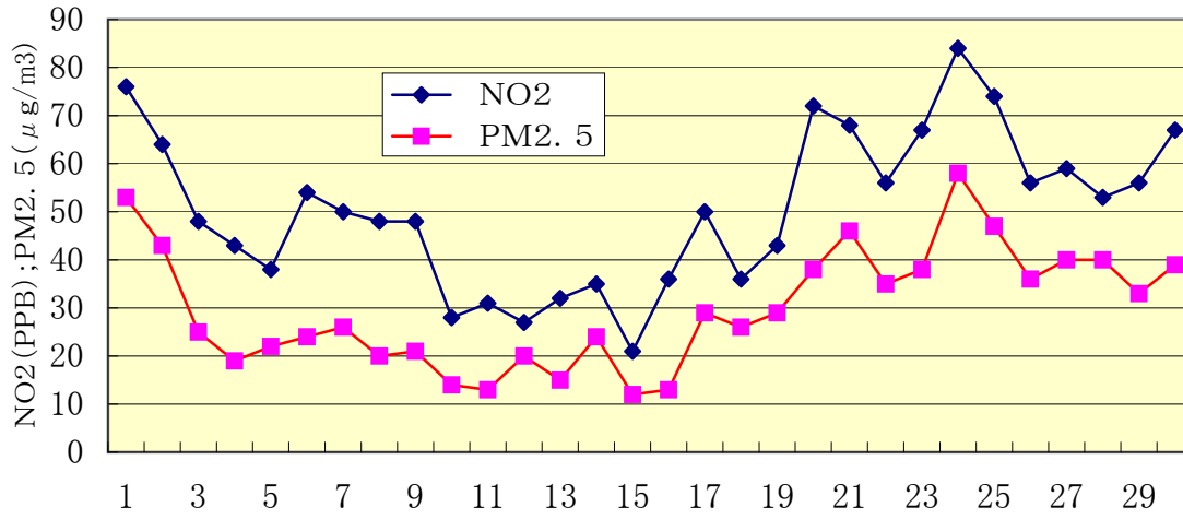
梅島自排局における日平均NO 2 とPM 2.5 の月間変動図 (2005年6月)
