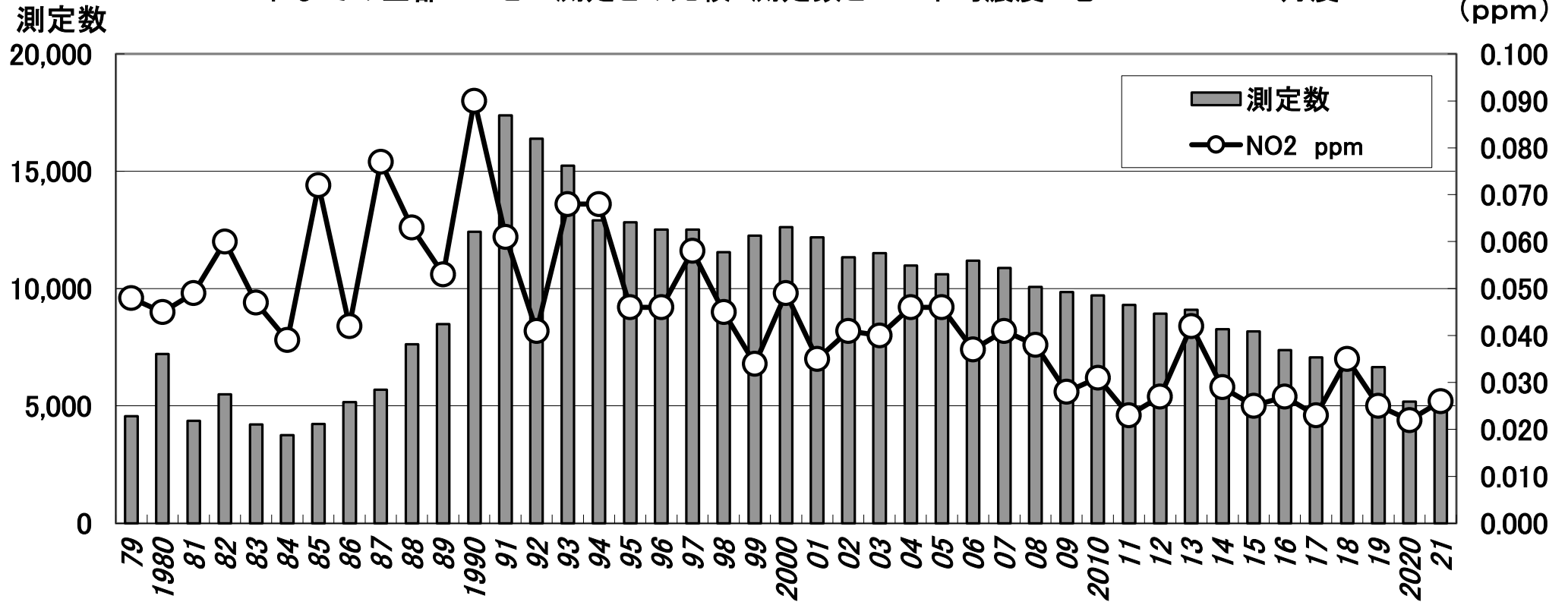
これまでの全都いっせい測定との比較 測定数とNO2平均濃度 地上1.5m 12月度
